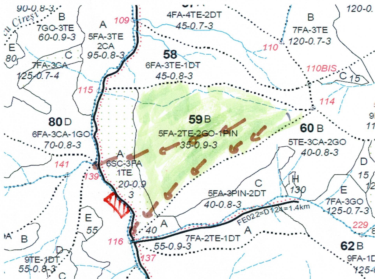
Coordonate GPS
